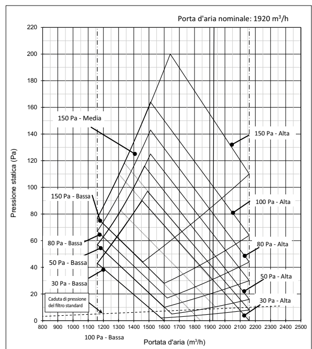
MMD-UP361BHP*
