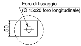
Dettagli dei piedini A
