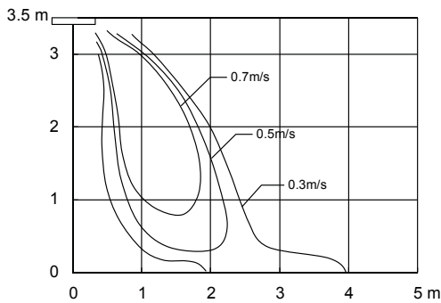
MMU-UP0151MH-E (modalità con soffitto alto)
