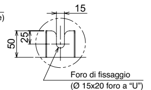
Dettagli dei piedini B
