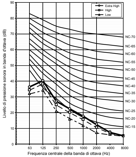
VN-M350HE
