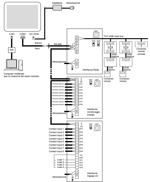
BMS-CT5121E
