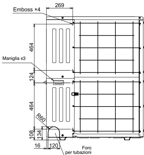
Foro pretranciato per la tubazione inferiore
