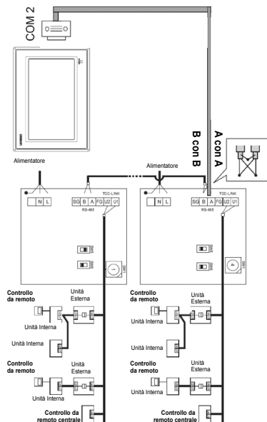
TCB-TSC640PY
