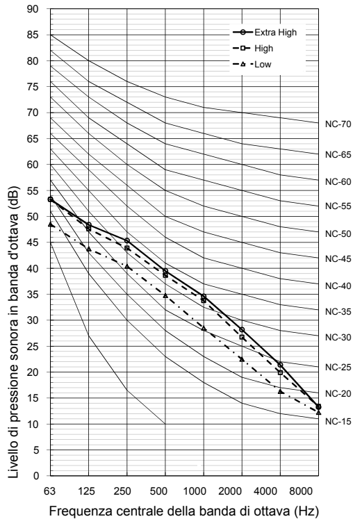
VN-M2000HE1
