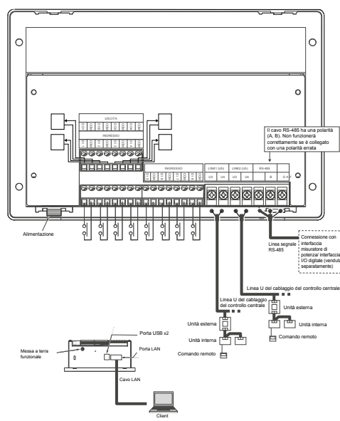
BMS-CT2560U-E
