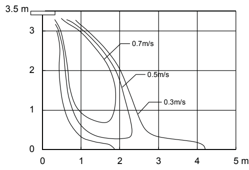
MMU-UP0181MH-E (modalità con soffitto alto)
