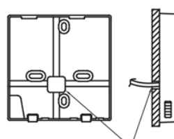
Foro nel muro e per i fili Diametro foro: Ø20mm
